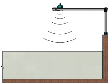
Figura 4: Suporte standard com 2 tubos
