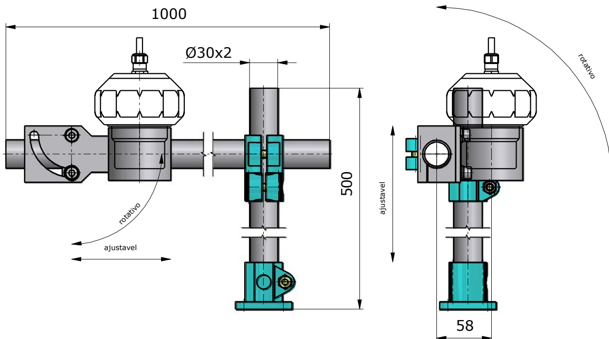
Figura 1: Suporte com Transmissor de Nível Ultrassônico
