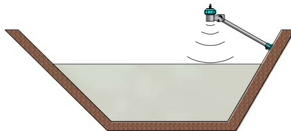
Figura 3: Montagem em bordas inclinadas
